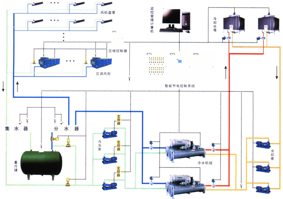
彩插 3 富士得水蓄冷智能节电控制系统
