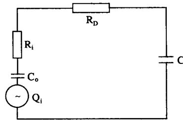
图 2-5 爆电法储电等效电路
