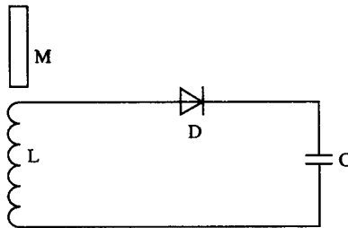
图 2-6 后坐发电机示意图
