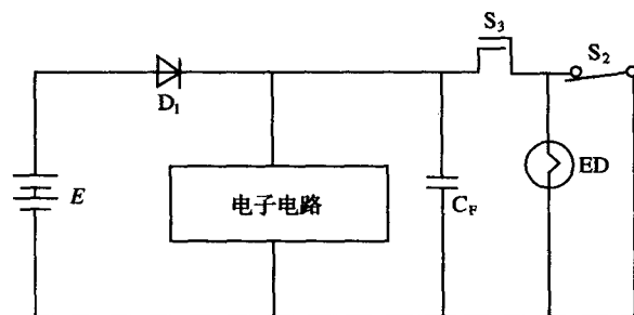
图 2-10 电源失效时发火保护电路
