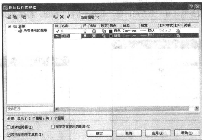
图 1-3 “图层特性管理器”对话框
