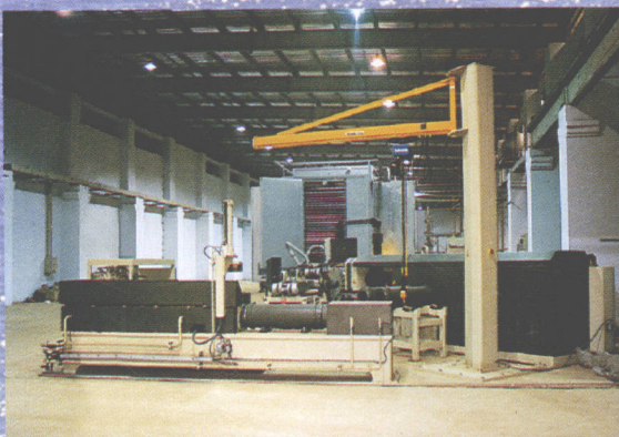
引进的德国贝尔纳公司电焊条生产线
