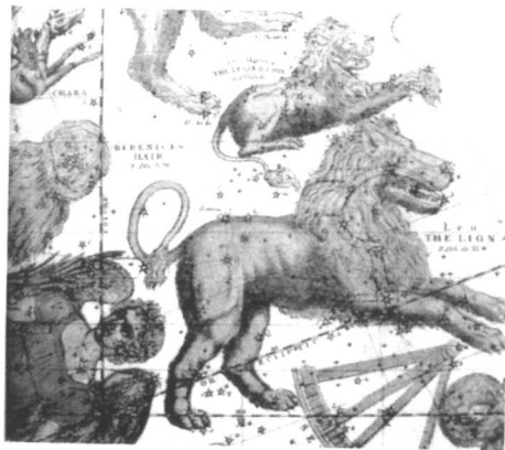
古典星图中的狮子座
