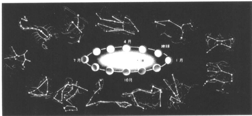
黄道十二星座
