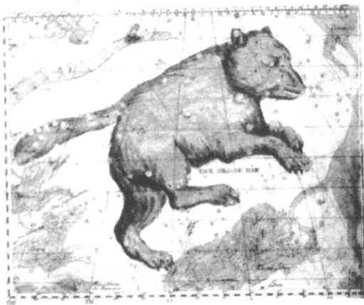
古典星相图中的大熊座
