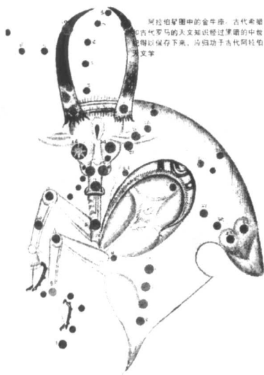
金牛座古典星相图
