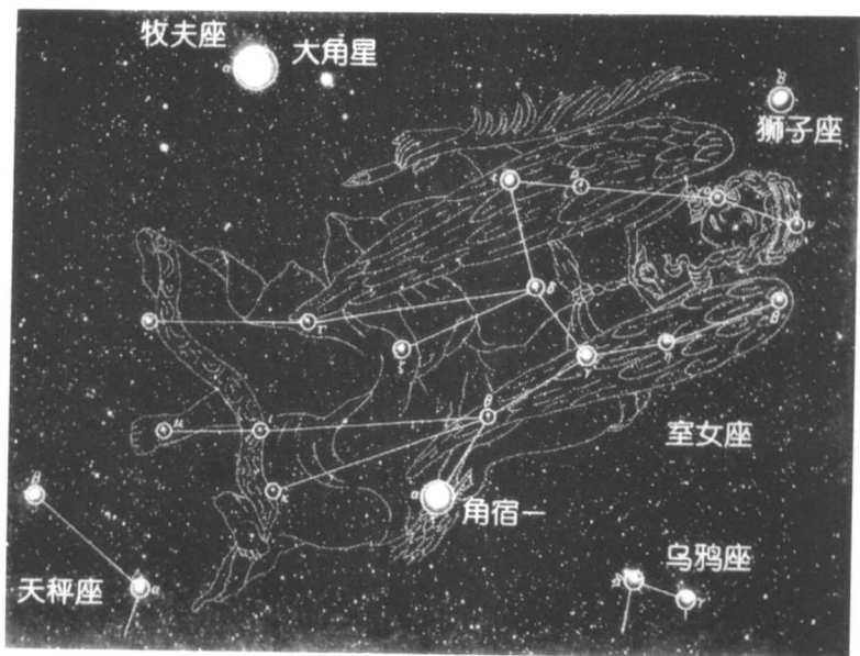
室女座的星图
