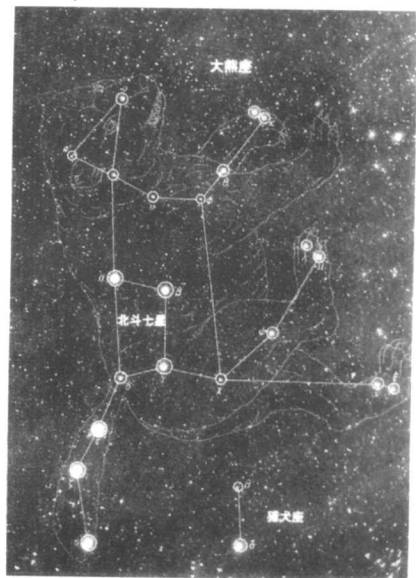
大熊座与北斗七星
