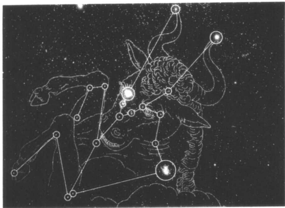
金牛星座星相图
