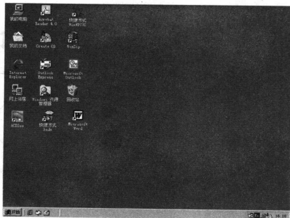
图 1-1 进入 Windows 98
