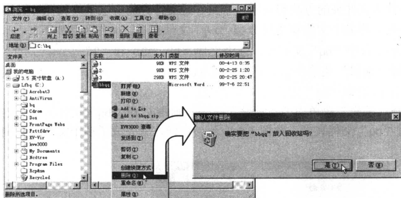
图 1-10 删除文件
