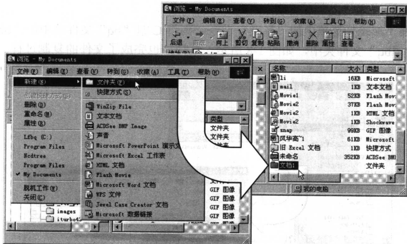
图 1-6 新建文件夹
