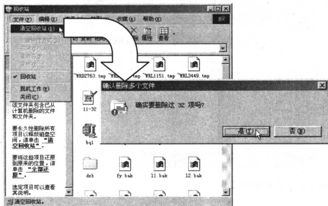
图 1-11 清空回收站
