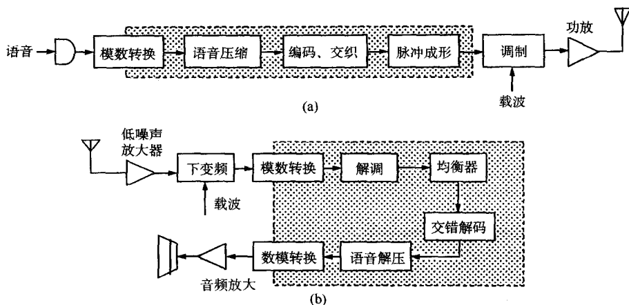
图 0.4 数字通信机的射频级电路方框图
