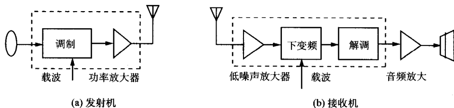
图 0.3 模拟通信机的射频级电路方框图
