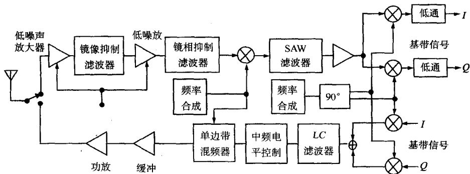
图 0.5 无线数字手机的射频级电路
