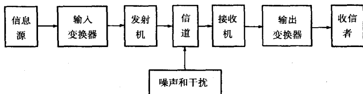
图 0.1 通信系统的基本组成
