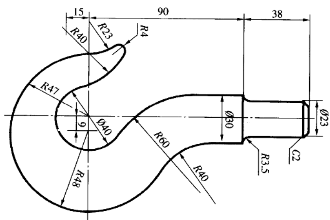
(2) 起重钩
