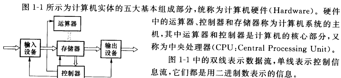
图 1-1 计算机的基本结构
