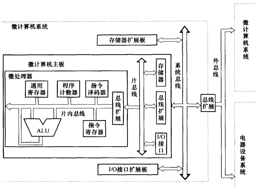
图 1-19 微型计算机的总线结构
