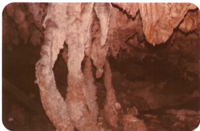
瑶兰洞 簇状石柱
