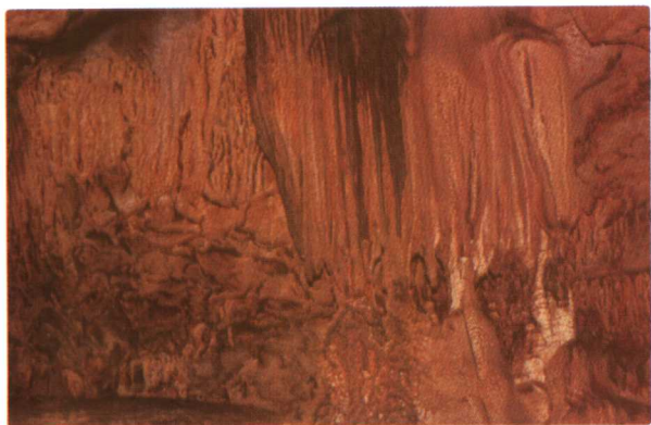
董歌洞 梯田状流石坝
