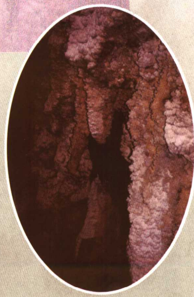
晶花状石钟乳
