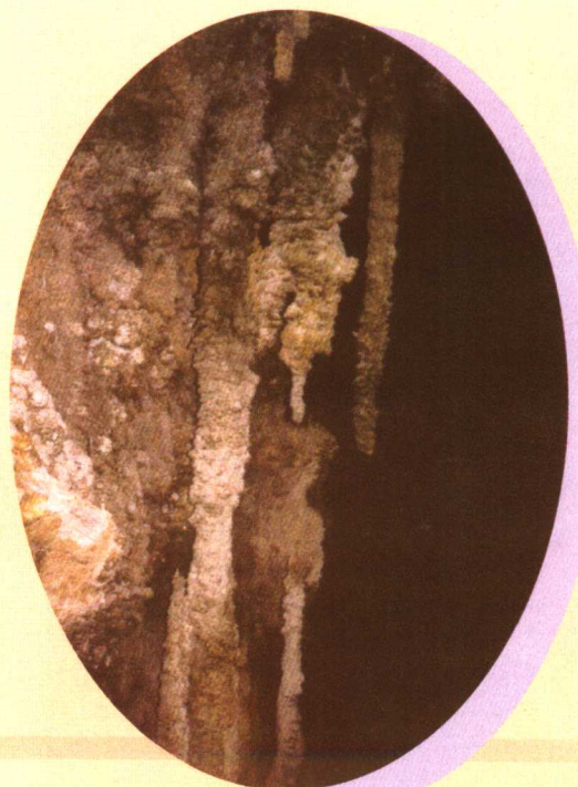
壁流石及石笋
