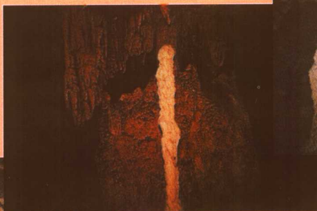
生长发生变化的石笋
