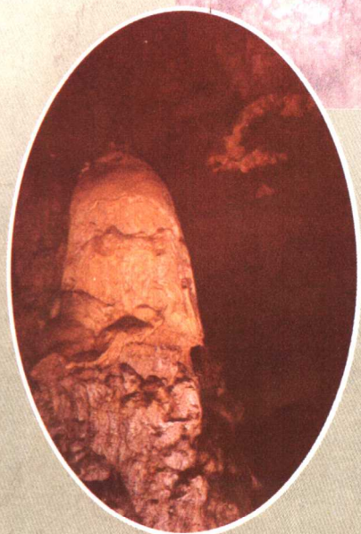
小七孔天钟洞 石钟
