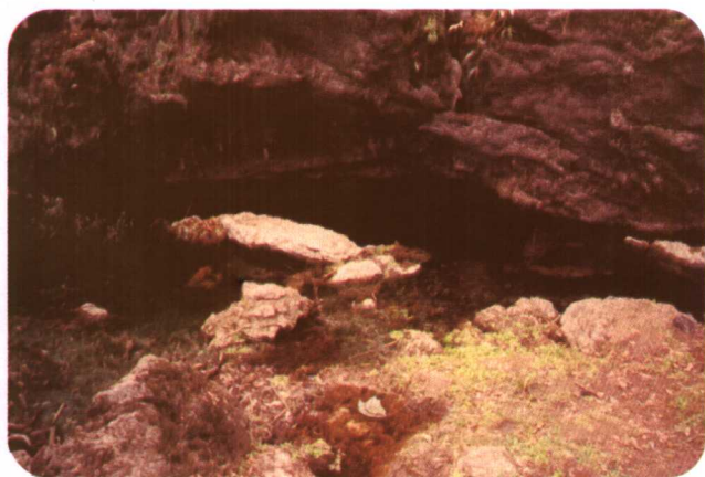
洞口的冲积物
