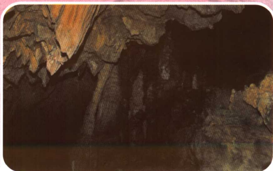
石旗与石笋的对应发育
