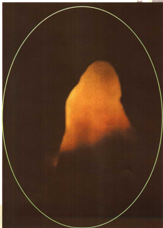
透明白色石笋
