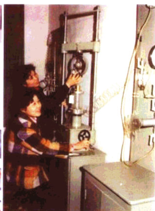
▲ 三轴剪力仪
