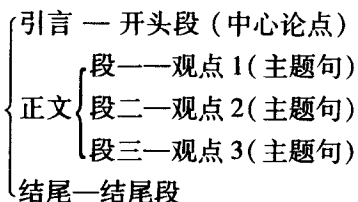
文章结构图
