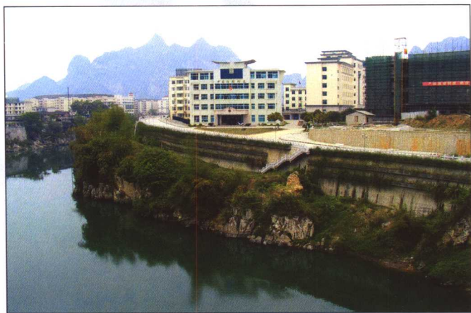
河池市龙江防洪堤堤景结合段
