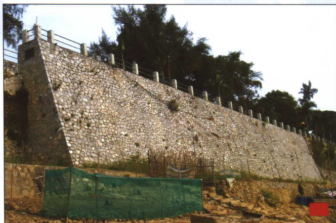
横县城防洪堤工程一角
