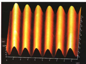
▼图5 用原子力显微镜获得的正弦相位光栅的浮雕轮廓
