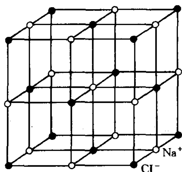
图 1-2 岩盐的内部构造
