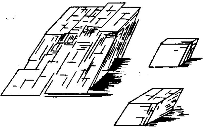
图 1-4 方解石的菱面体解理
