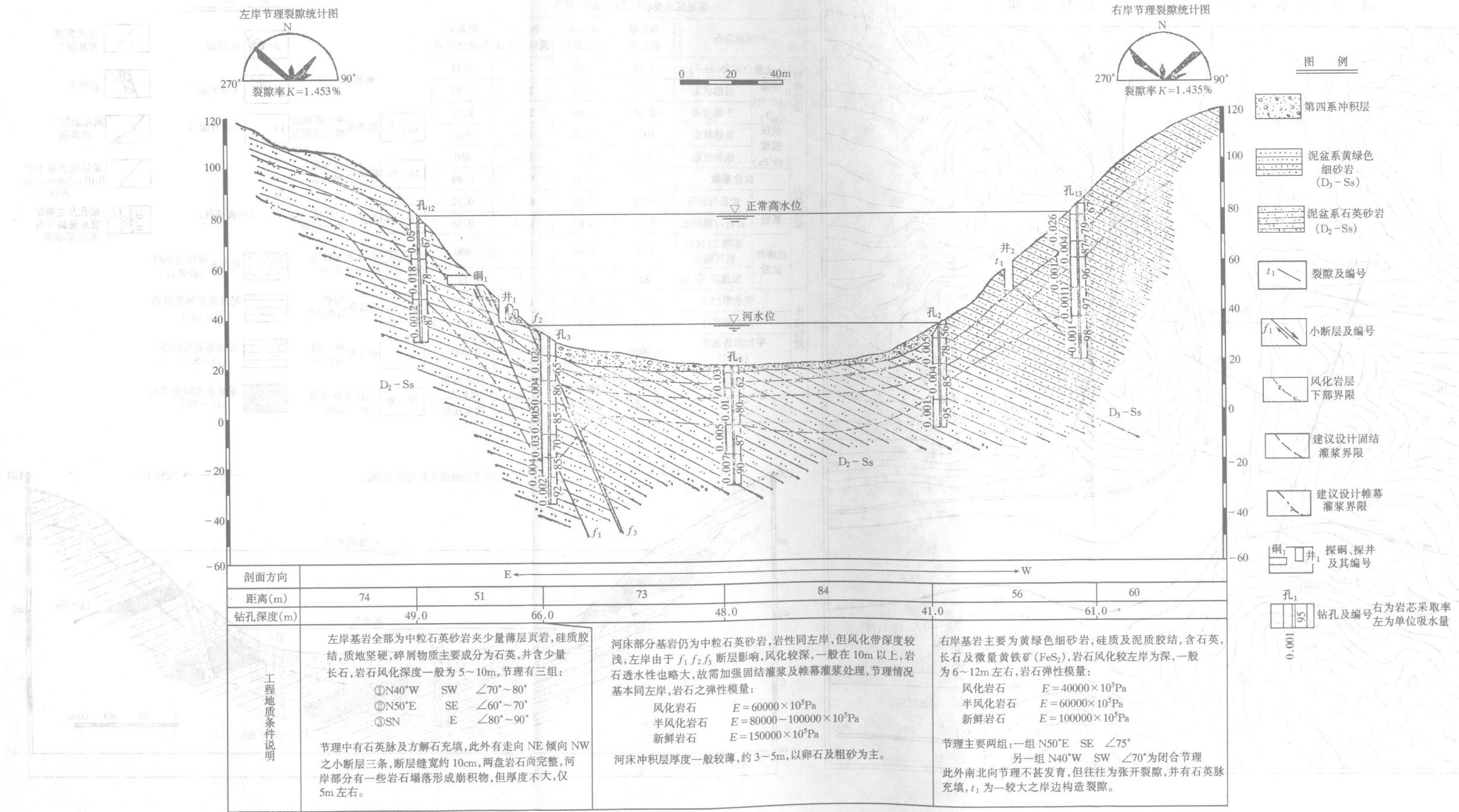
梅村坝址 第一坝轴线专门性工程地质剖面图
