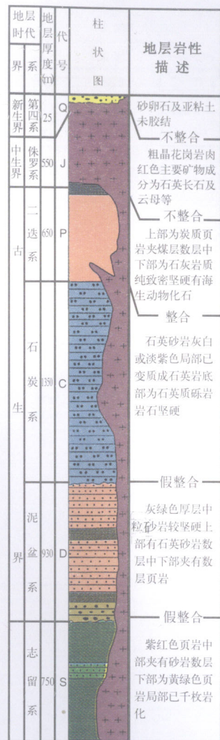
地层柱状图
