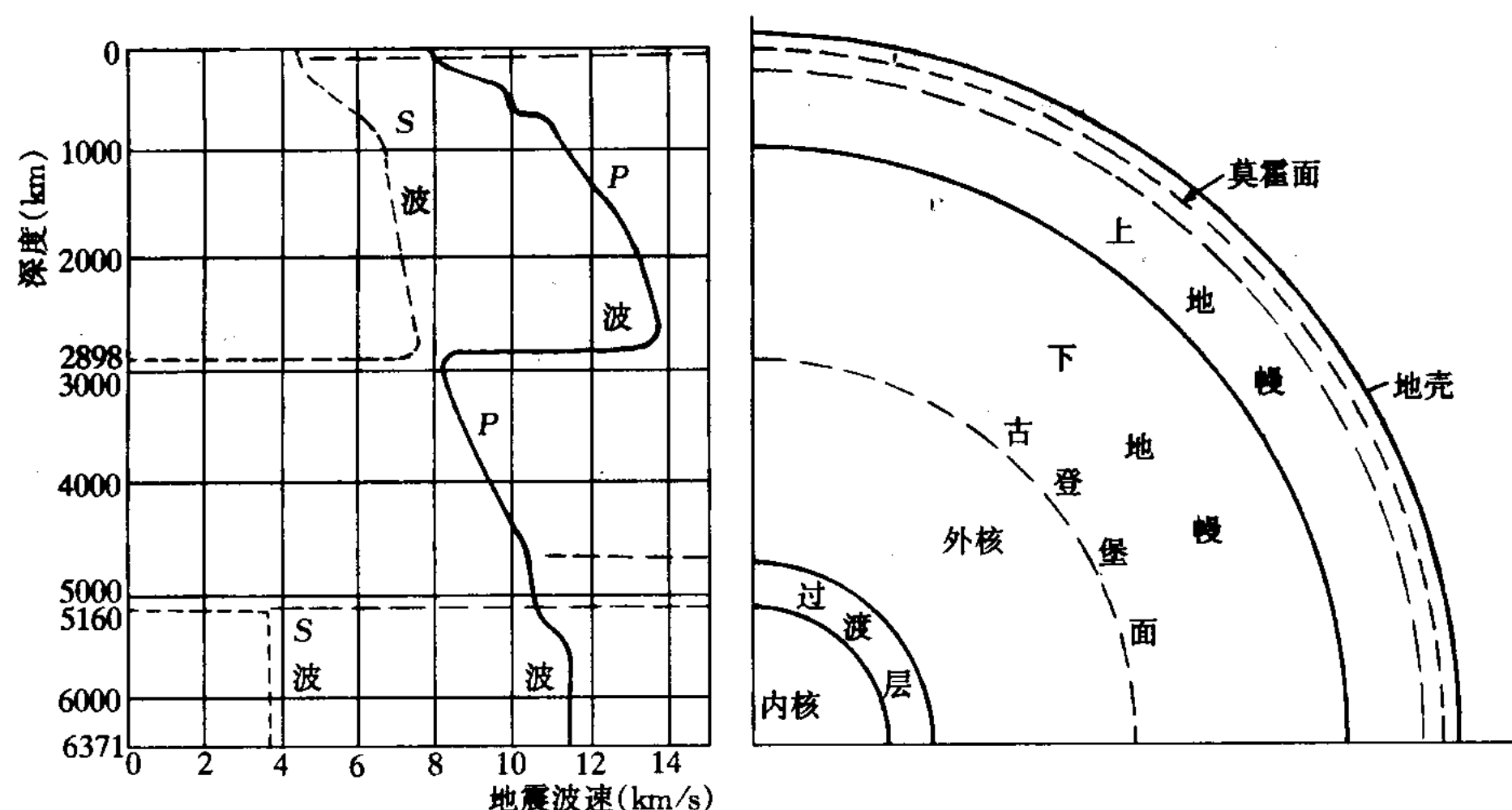
图 1-1 地球内部结构图
