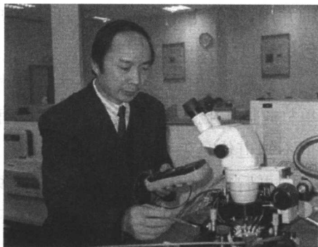
王志功在研究所
