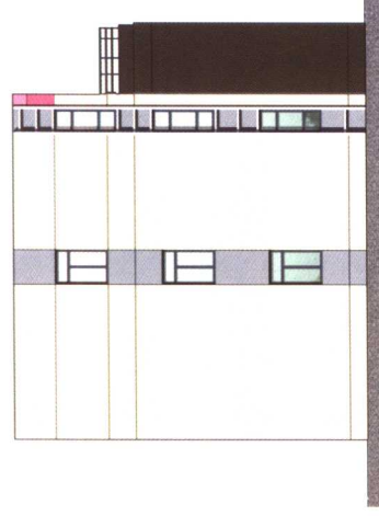
西立面图 1: 200
