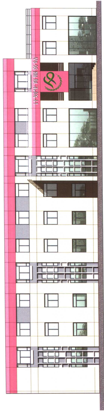
南立面图 1: 200
