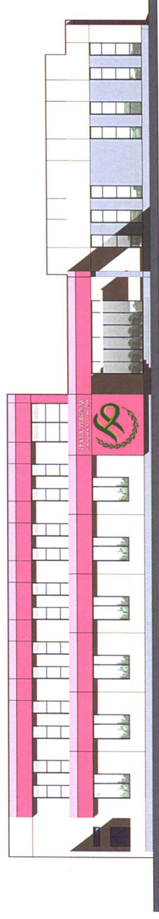
南立面图 1: 200
