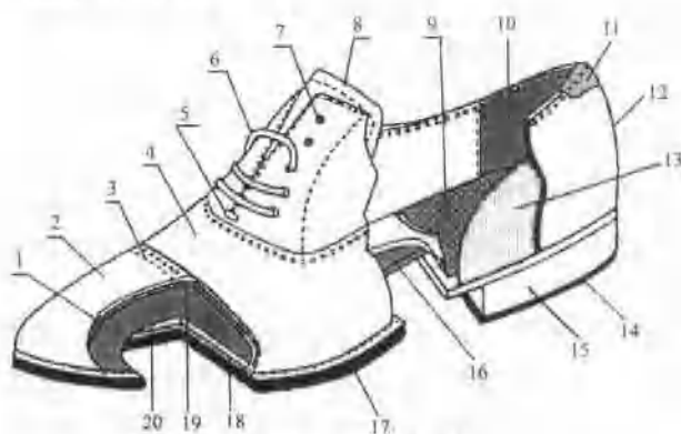
图 0-1 鞋的零部件
