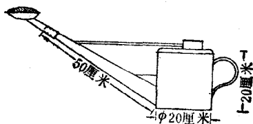
图1 活头细眼喷壶示意图
