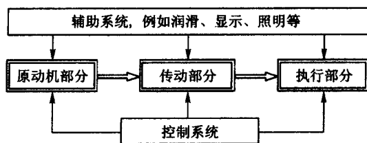
图 2-1 机器的组成
