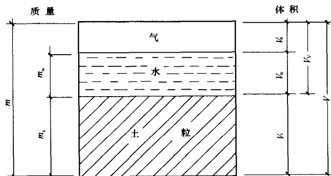
图 1-4 土的三相组成示意图
