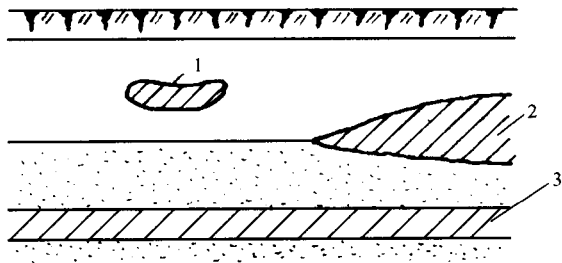
图 1-1 土的层理构造
