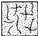
图 1-2 裂隙构造
