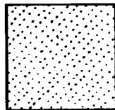
图 1-3 分散构造
