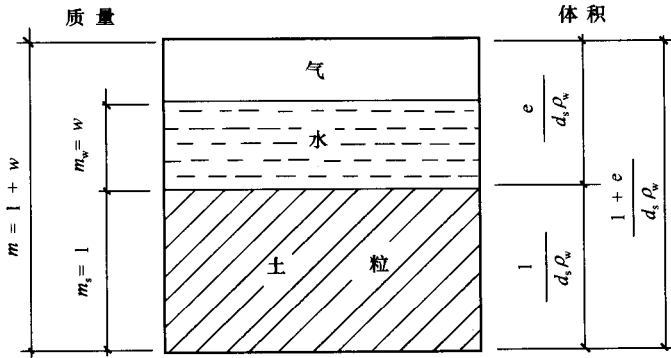
图 1-5 土的三相物理指标换算图
