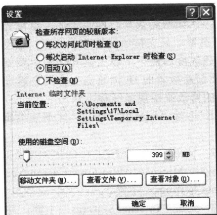
图 1-1-4 【设置】对话框
