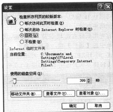
图 1-1-6 【设置】对话框
