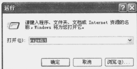
图 1-1-1 【运行】对话框
