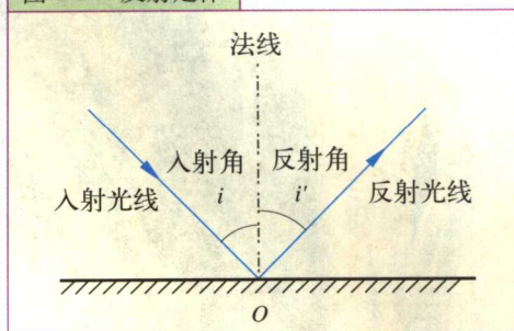
图 1.1-2 反射定律
