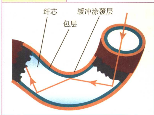
图 1.2-5 光纤结构
