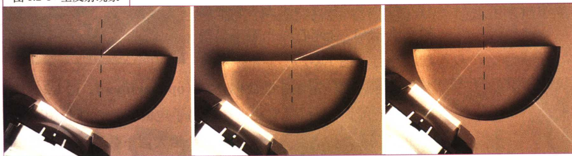
图 1.2-1 全反射现象
