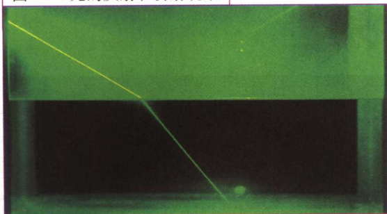
图 1.1-1 光的反射和折射现象
