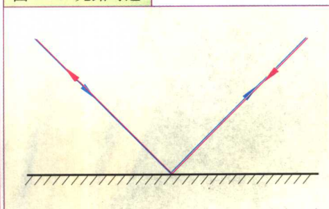
图 1.1-3 光路可逆
