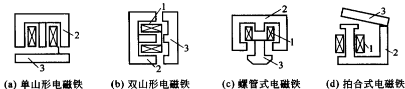
图 1-1 电磁机构的几种结构形式
