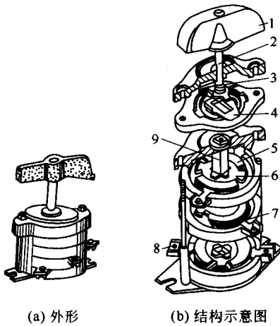
图 1-15 HZ10 系列组合开关
