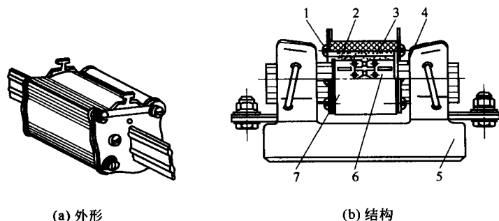
图 1-12 RT0 系列有填料封闭管式熔断器
