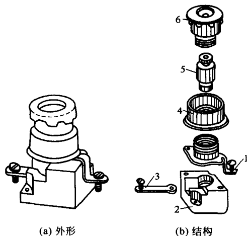
图 1-10 RL1 系列螺旋式熔断器
