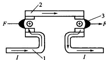
1-4 双断口结构的电动力吹弧效应 1—静触头；2—动触头；3—电弧
