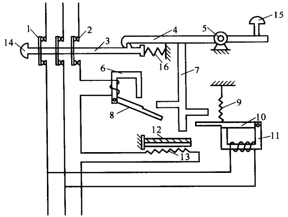
图 1-16 自动空气开关原理示意图
