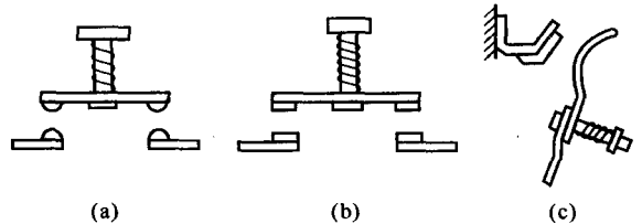
图 1-3 触头的结构形式
