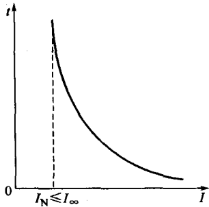
图 1-8 熔断器的安秒特性
