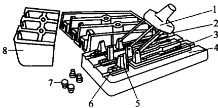
图 1-14 HK2 系列瓷底胶盖刀开关
