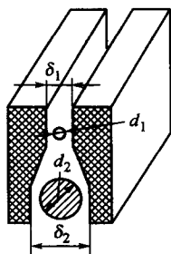
图 1-5 窄缝灭弧室的断面
