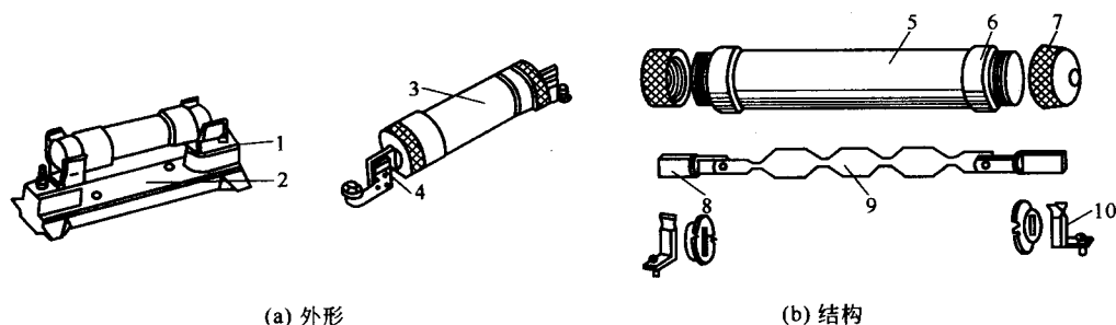
图 1-11 RM10 系列无填料封闭管式熔断器
