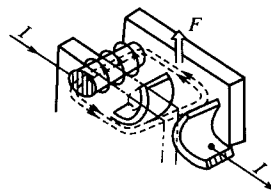
图 1-7 磁吹灭弧
