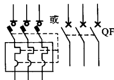
图 1-18 自动开关的图形和文字符号
