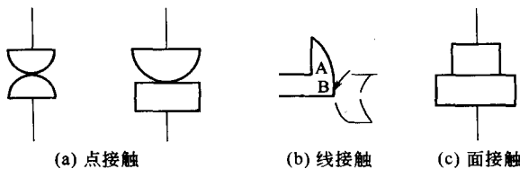
图 1-2 触头的三种接触形式
