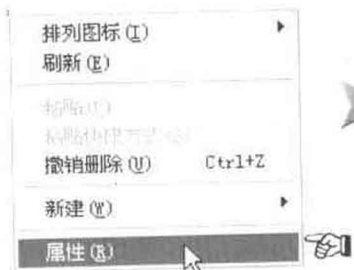
图 1-29 选“属性”命令
