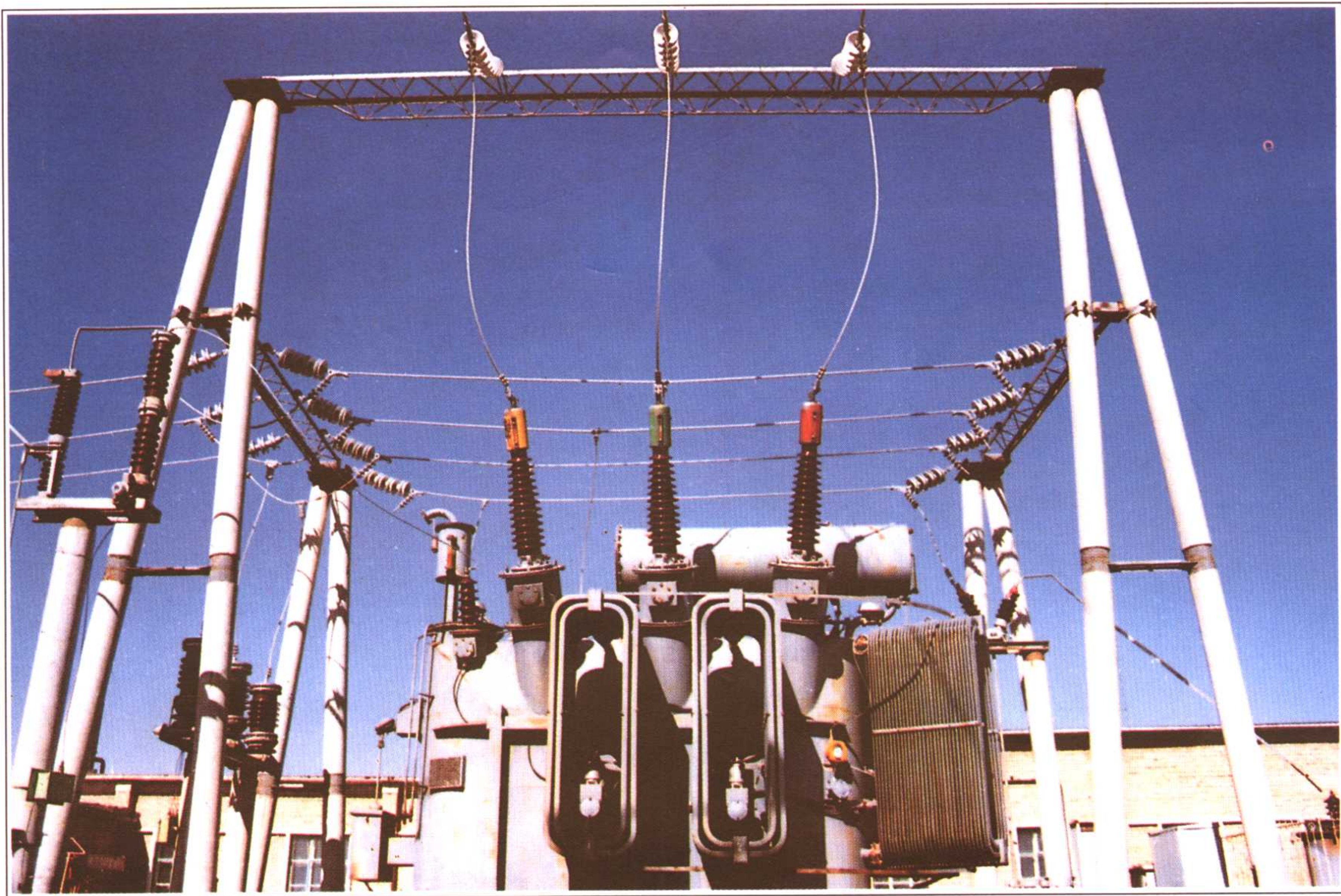
黄脑包 110 千伏变电站
