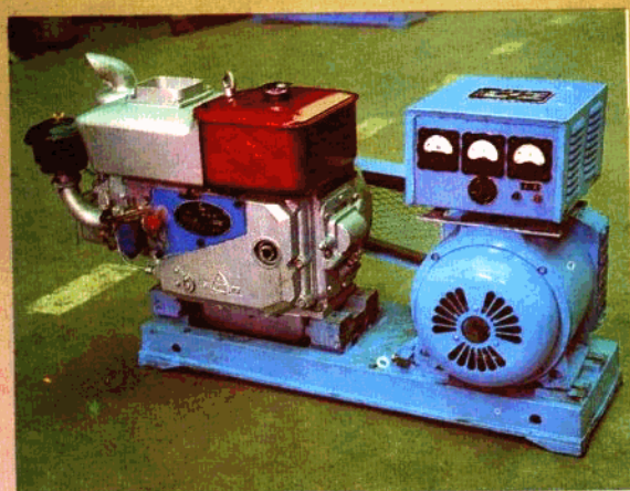
7.5KW柴油发电机组
