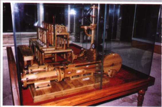
陈启沅设计的机器缫丝机模型图。
