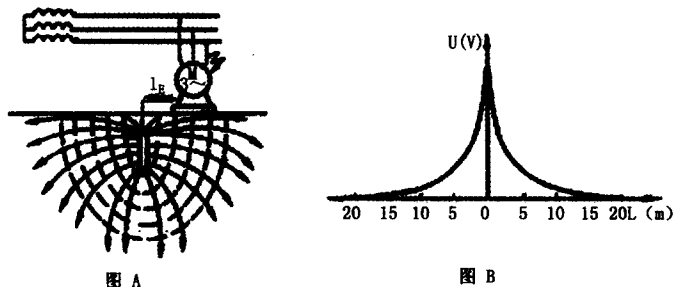
图 1-3 地中电流的流散电场和地面电位分布
