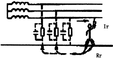
图 1-1B 中性点不接地电网
