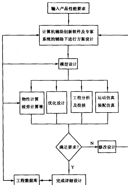
图 1.1 机械 CAD 设计过程
