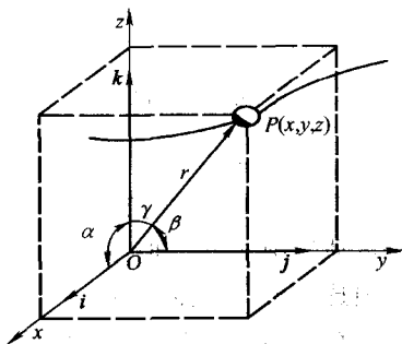
图 1-1 位置矢量
