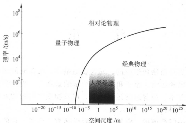
图 0-2 不同时空尺度和速度
