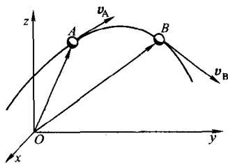
图 1-4 速度的变化
