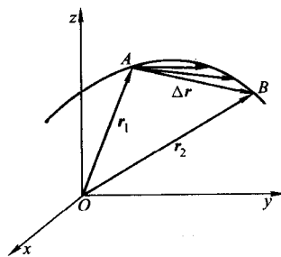
图 1-3 质点的速度
