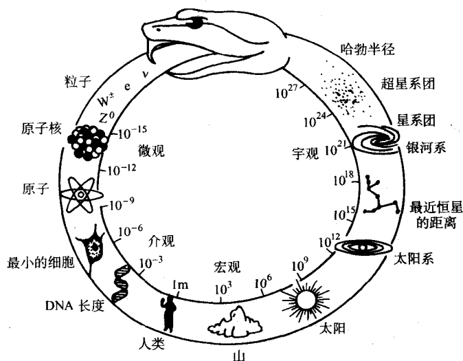
图 0-3 物理学大蟒蛇
