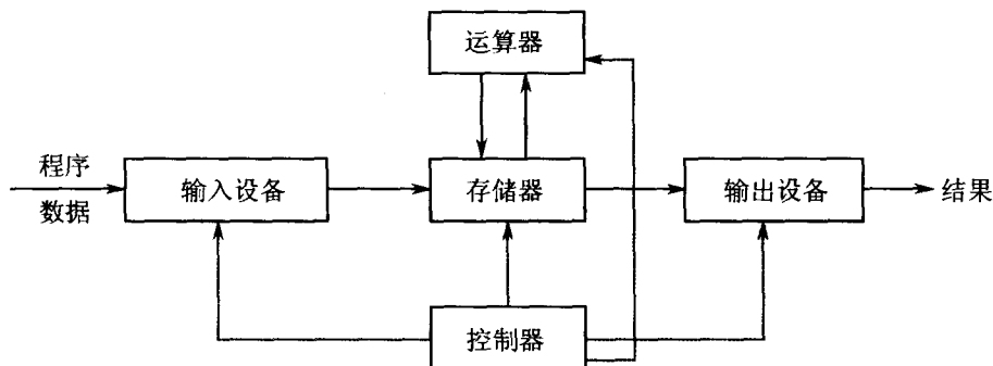
图 1-3-2 冯·诺依曼结构体系
