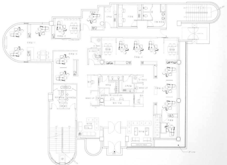
1楼平面图
