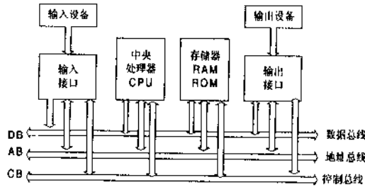
图 2-1 微型机总线结构
