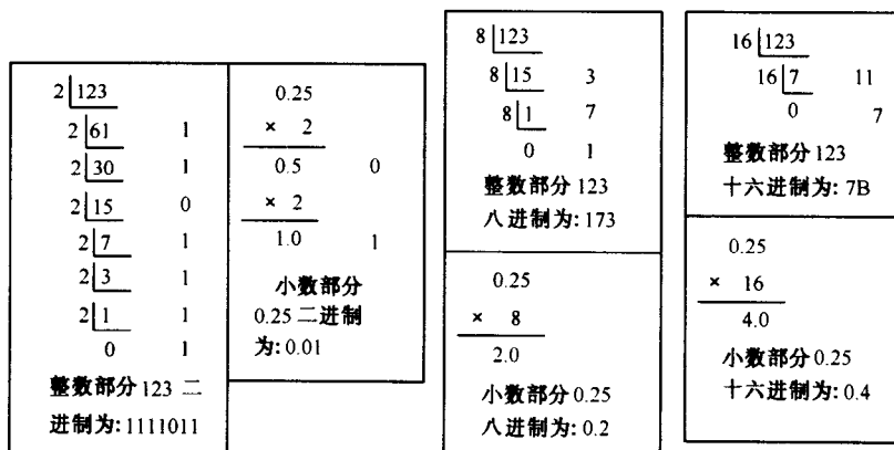
图 1.3 十进制转换为其他进制的一般方法
