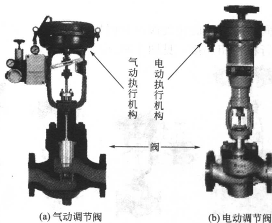
图 1-7 调节阀
