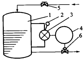
图 1-5 人工控制液位示意图 1—液体储槽；2—显示仪表；3—液位变送器； 4—调节器；5—入口阀门；6—调节阀
