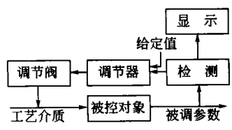
图 1-6 方块图
