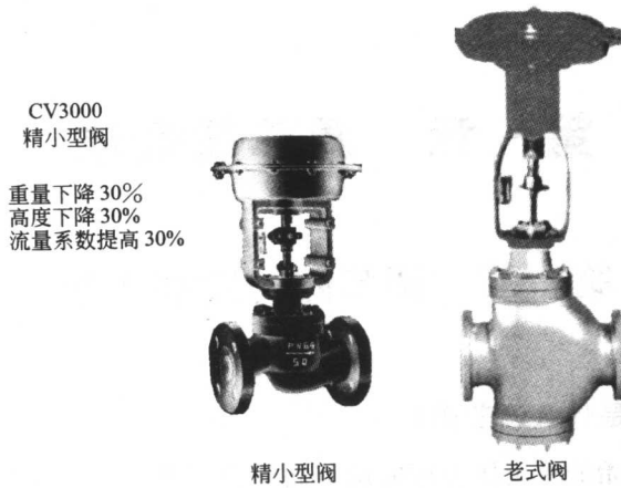
图 1-1 CV3000 精小型阀与典型老式阀的比较
