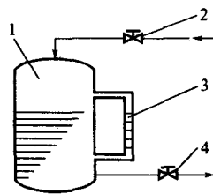
图 1-4 人工控制液位示意图
