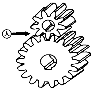
图 1—1 齿轮传动
