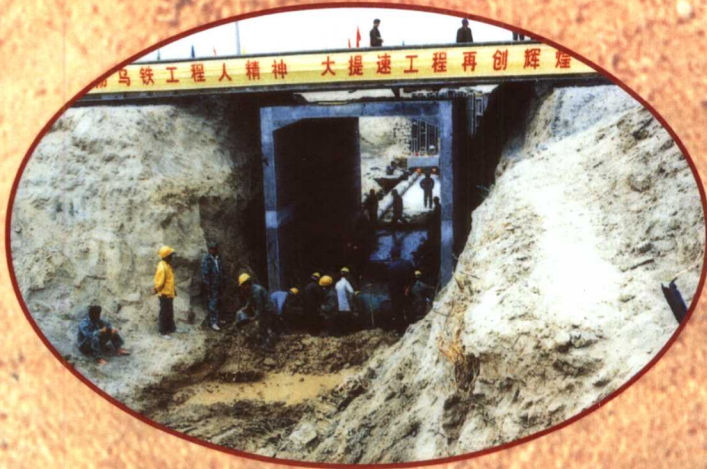
二段提速施工顶进桥涵
