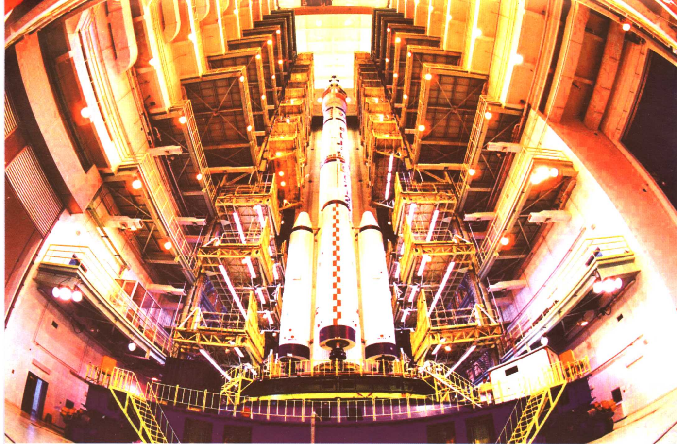
▲ CZ-2F 在垂直测试厂房
