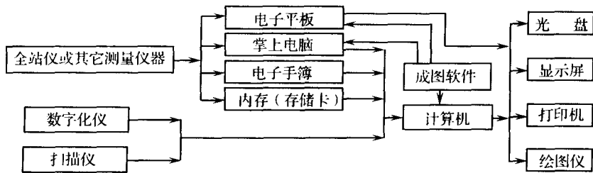
图 1-4 数字测图系统流程示意
