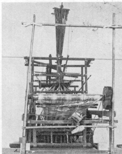
清嘉庆、 道光年间，四 川成都机房制 作的蜀锦机。 织锦时，需要 二人配合，一 人纬丝，一人 提花。
