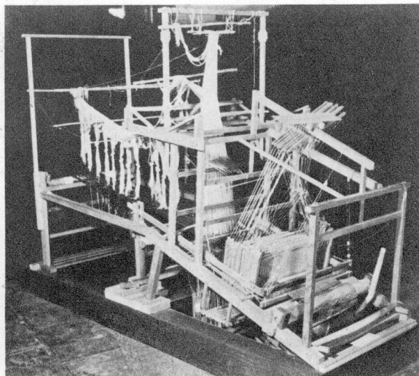
南京旧机业公所 织缎机。
