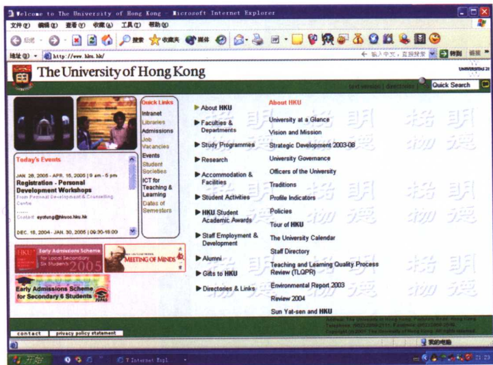
图 1.1 典型主页
