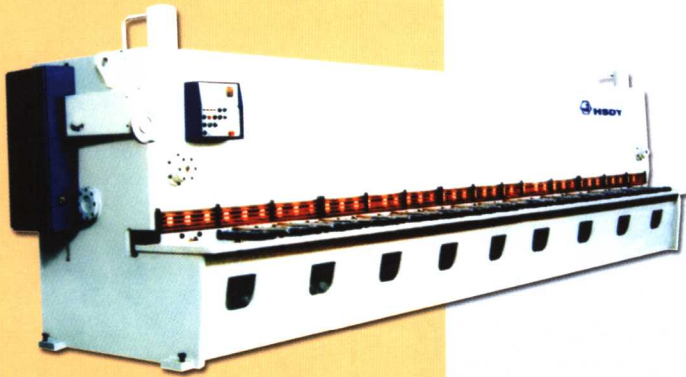
液压(数控)剪板机 (闸式) 引进比利时LVD技术) HGA(K)HGO(K)HGN(K)HGS(K) 系列 最大剪切厚度 40mm \sigma_b \leq 450 MPa 最大剪切长度 16000mm
