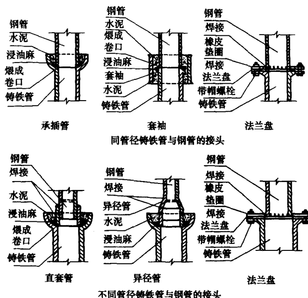
图 2.4.4-2 给水铸铁管与镀锌钢管连接方法
