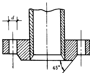
图 2.4.4-4 法兰盘
