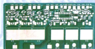
铝基板
