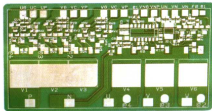
铝基板
