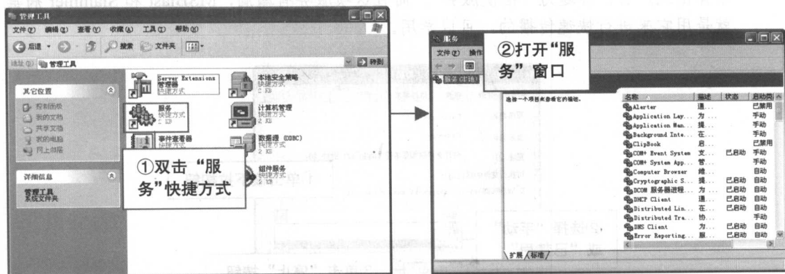
图 1-7 “服务”窗口
