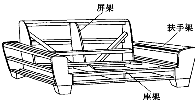
图 1-5 双位沙发木架结构
