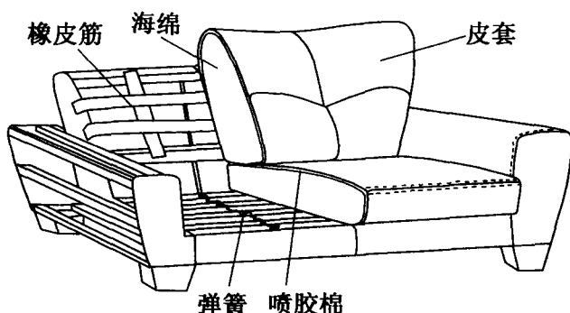
图 1-4 双位沙发内部结构
