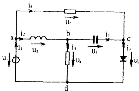
图 16-1 表示基尔霍夫定律的电路图示
