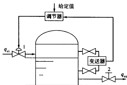
图 1-2 贮罐液位的自动控制系统示意图 1—执行器；2—出料阀
