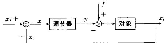
图 1-11 定值控制系统的方框图
