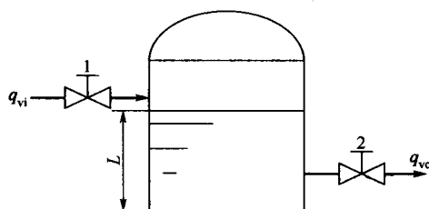
图 1-1 贮罐液位的手动控制系统示意图 1—进料阀；2—出料阀
