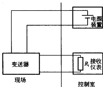
图 1-6 变送器的四线制传输
