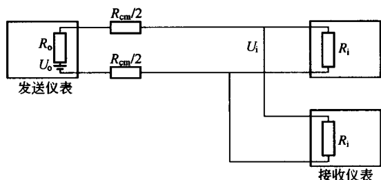
图 1-5 直流电压信号传输时仪表之间的连接
