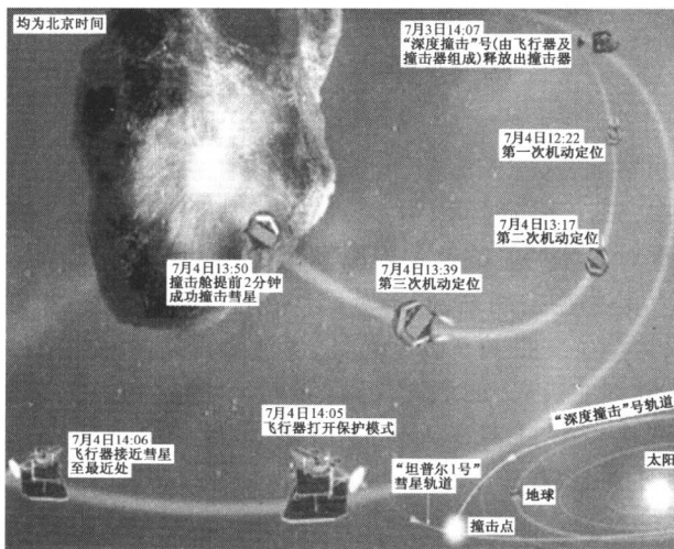
图1-4 “深度撞击”示意图
